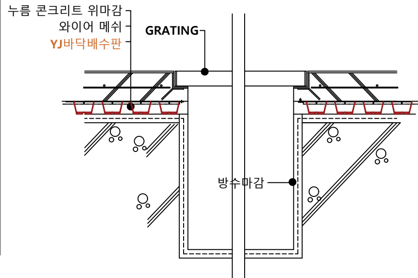
집수정 상세도
