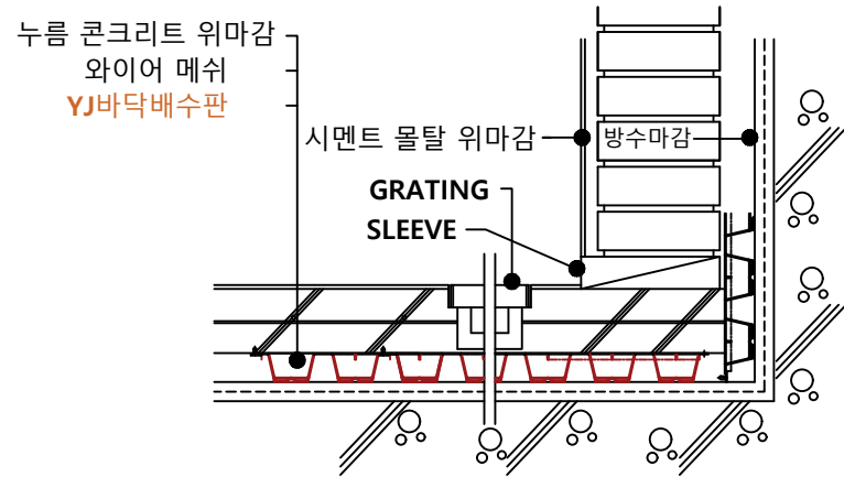
트렌치 상세도
