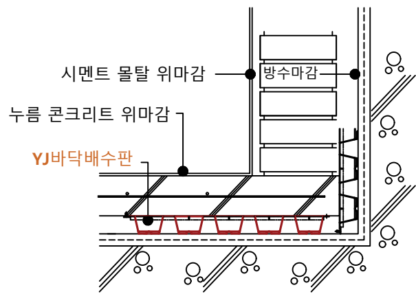
배수 보호벽 상세도
